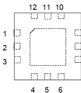
&lt;Top View&gt;
