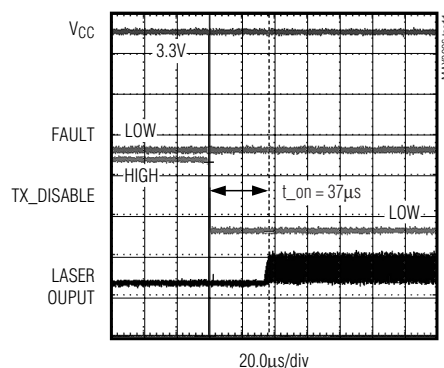
TRANSMITTER ENABLE
