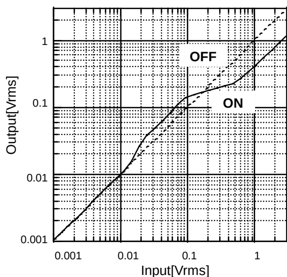
AGC
