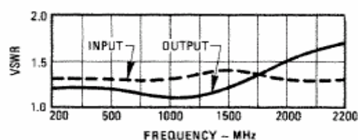
VSWR
