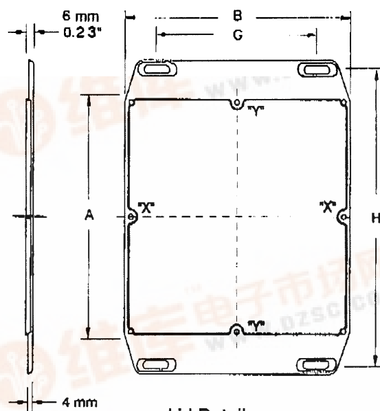
Lid Detail
