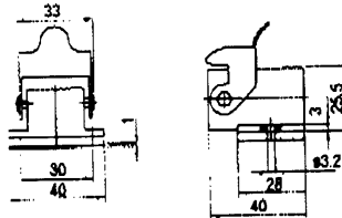
Montageausschnitt/Panel cut-out ø 20
