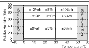
■ Feuchtesensor 9701 – Genauigkeit
