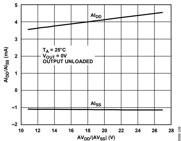
Figure 8. A_{Le}/A_{Iss} vs. AV_{DD}/AV_{SS}
