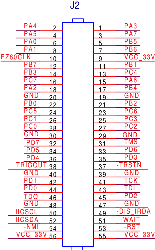
Figure 3. eZ80F91 Mini Enet Module I/O Mini Module Connector Pin Configuration—J2
