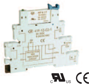
Montaje en Riel DIN.
