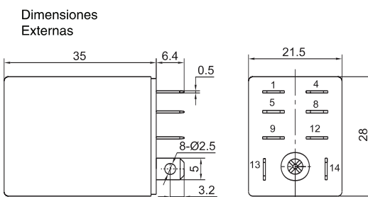
Serie RL1/RL2
