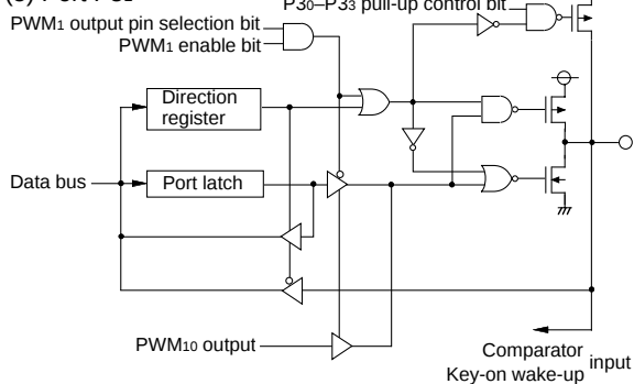
(5) Port P31
