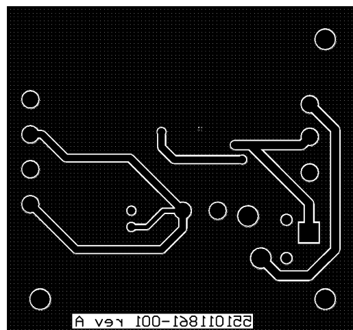
Bottom Layer
