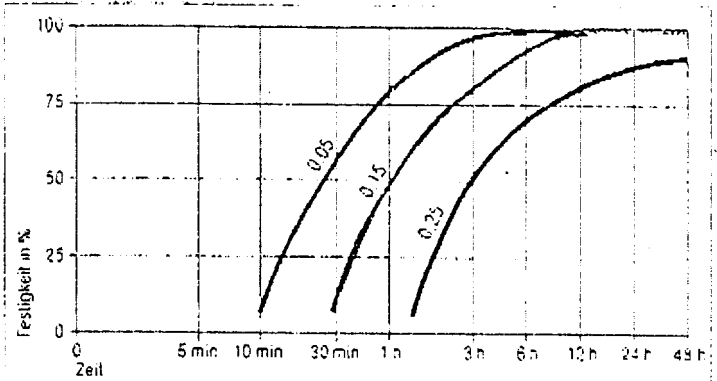
Aushärtung mit Aktivator an gelbchromatierten Teilen Test in Anlehnung an DIN 54454
