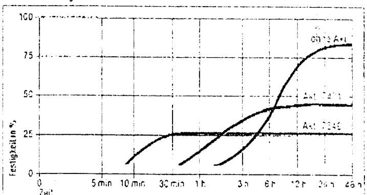
Wärmealterung Test in Anlehnung an DIN 54454
