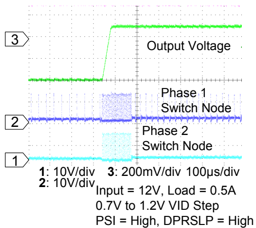
Figure 18. VID Step
