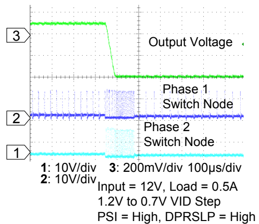
Figure 17. VID Step
