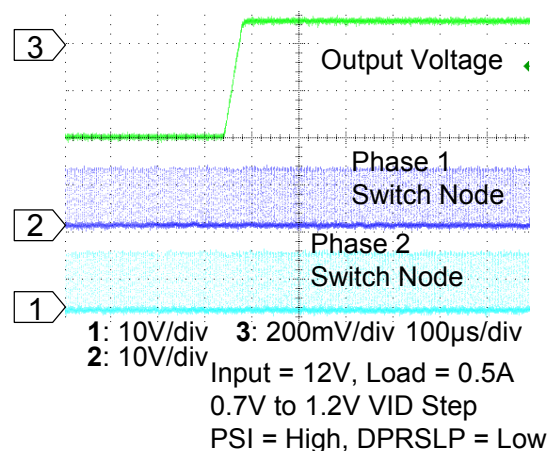
Figure 20. VID Step
