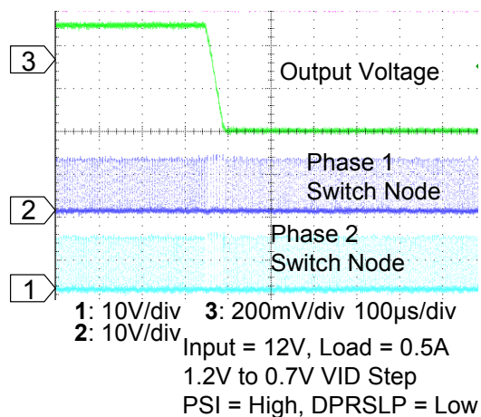
Figure 19. VID Step
