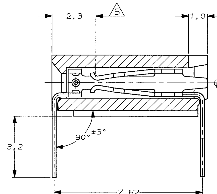
SECTION A-A
