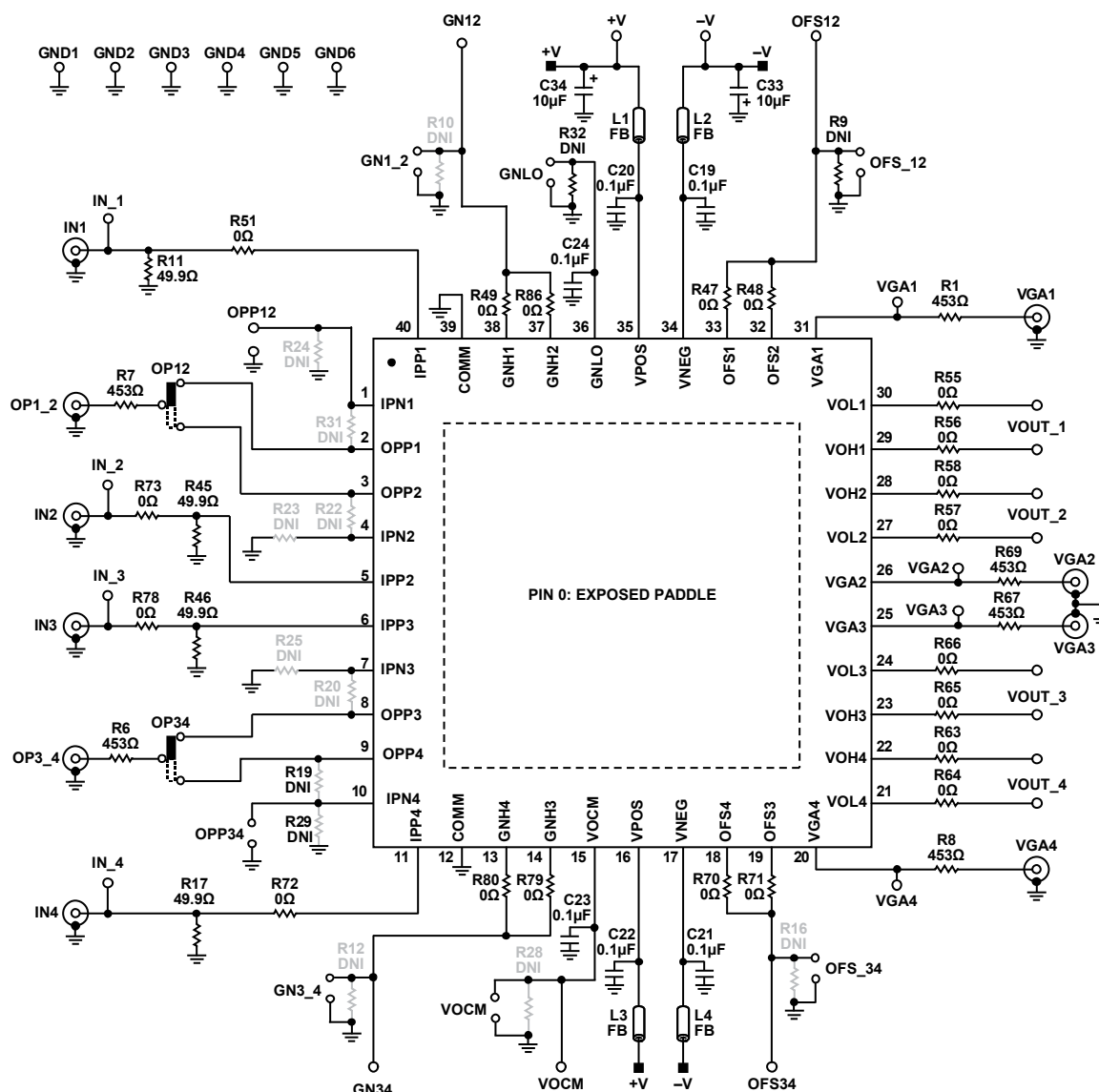
Figure 118. AD8264-EVALZ Schematic
