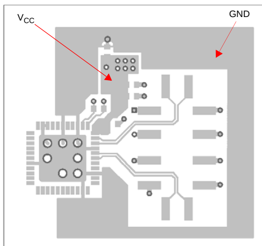
Figure 30: IF part: top layer
