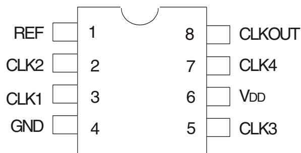
SOIC/TSSOP TOP VIEW
