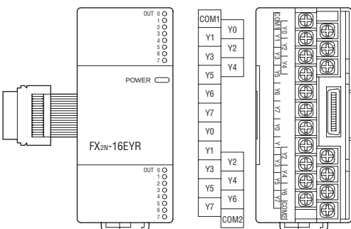
FX2N-16EYR-ES/UL
