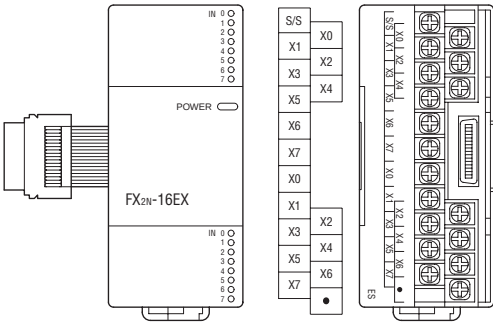
FX2N-16EX-ES/UL
