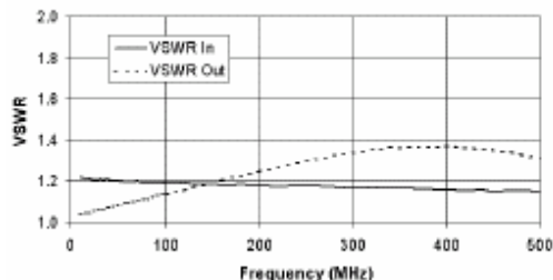
VSWR
