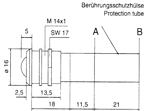
Schnitt / cut A - B
