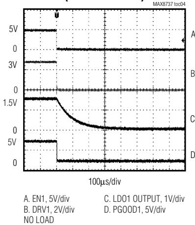
SOFT-STOP (EN FALLING EDGE)
